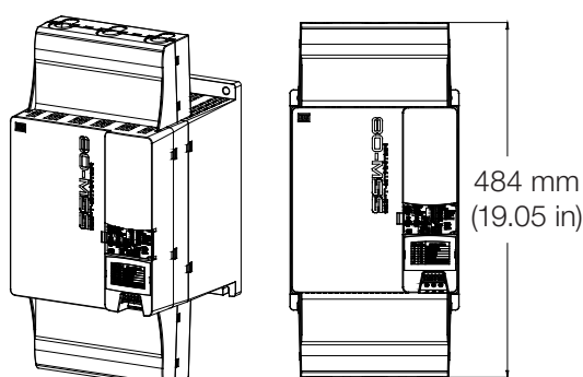
Figura 7.2: Kit IP20 para mecânica 4
