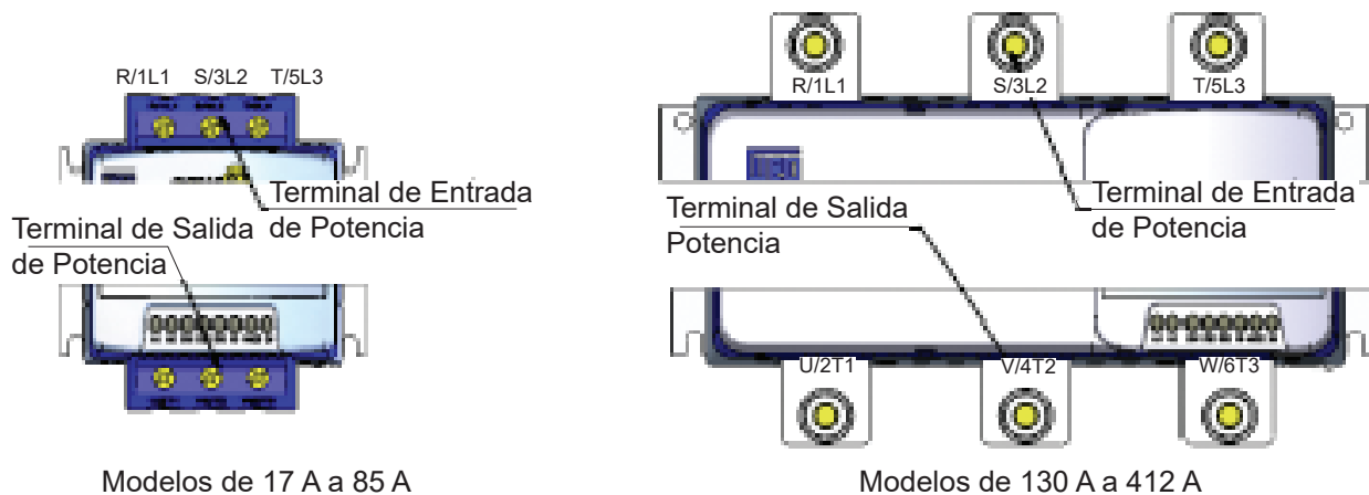
Figura 3.5: Terminales de potencia
